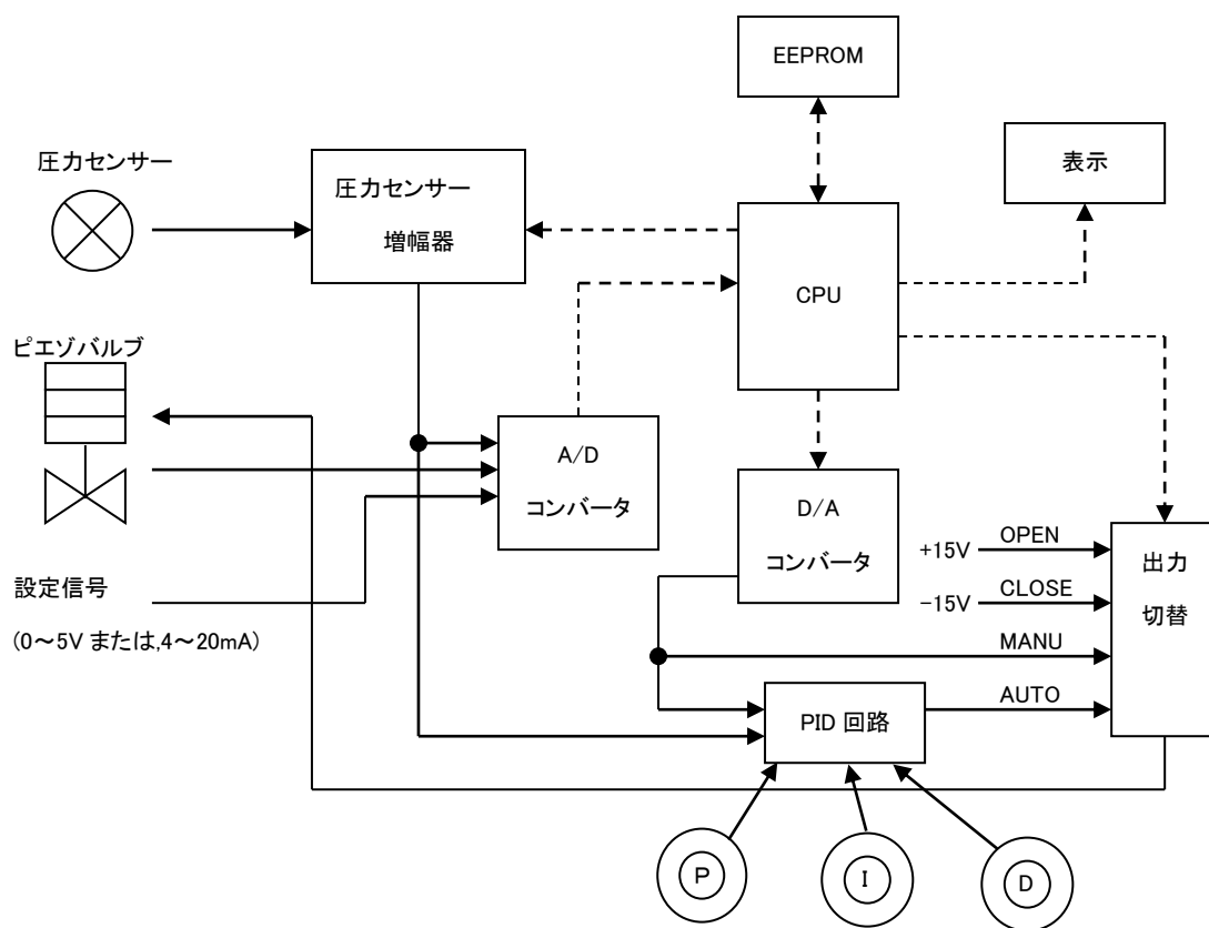
(ブロック図)
